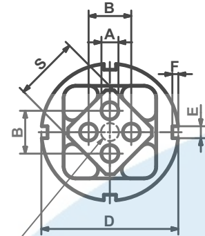
DK-A 50: \varnothing 20^{+0.5}
