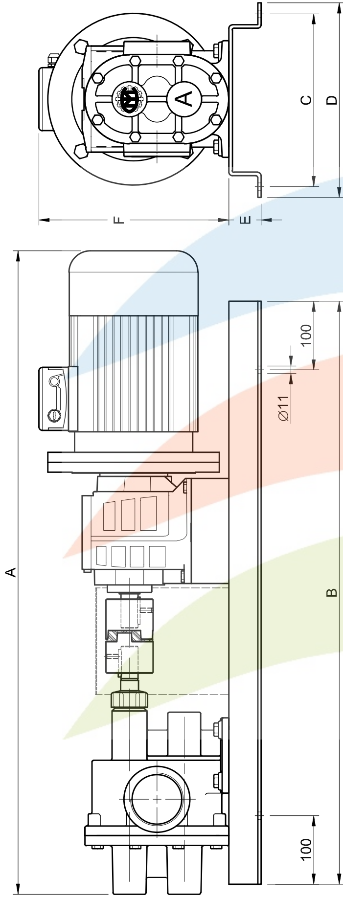
Datos dimensionales / Dimensional data
