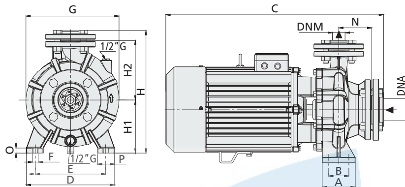
Flange Flanges
