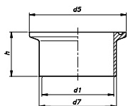
CASQUILLO CLAMP SOLDAR WELDING CLAMP FERRULE CLAMP À SOUDER
